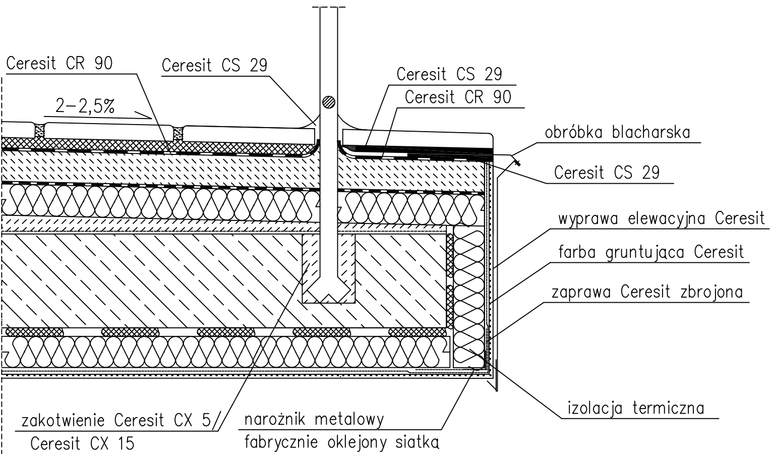
Rys. 9 - Krawędź okapu balkonu ocieplonego
